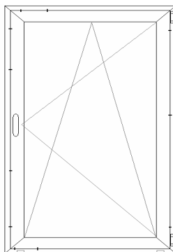
960 x 2210 mm
